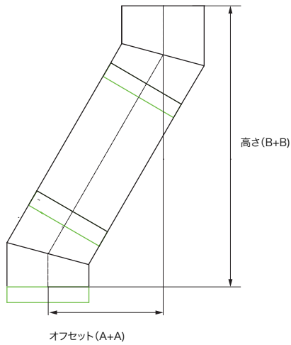
曲がりの構成例(エルボ+直筒)
