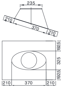
瓦用鉛フラッシング (5~30°勾配)
