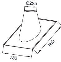
SUS板フラッシング 5~30°勾配用
