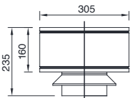
丸トップ 壁出し専用
