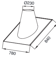
30~45°勾配用
