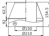
角トップアダプター
